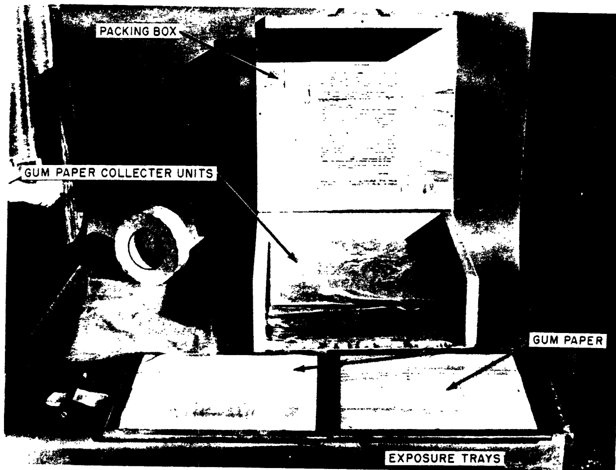
Fig. 3.7—Gum-paper collector kit.
