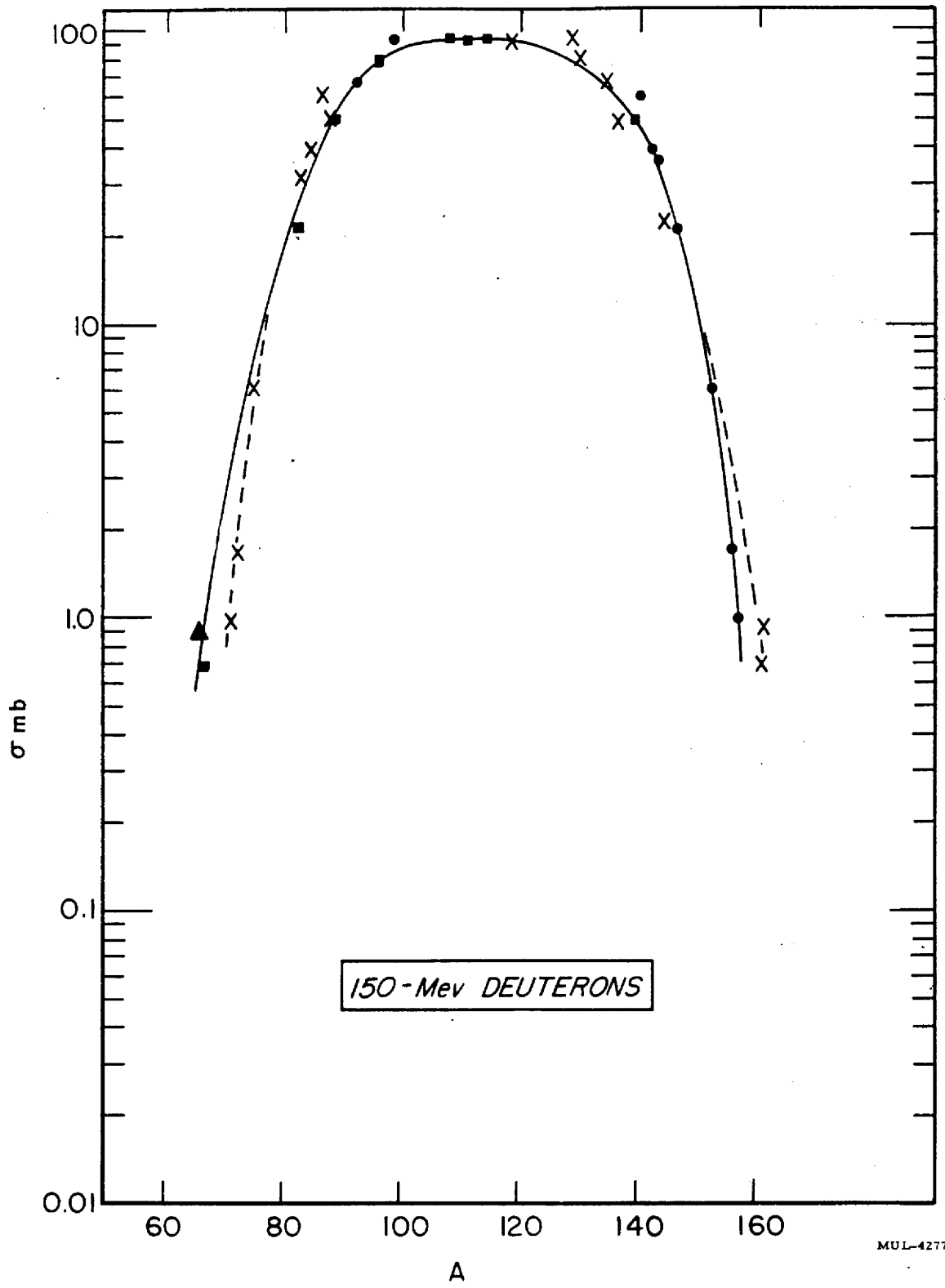
Fig. 2 F. 150-Mev Deuterons
