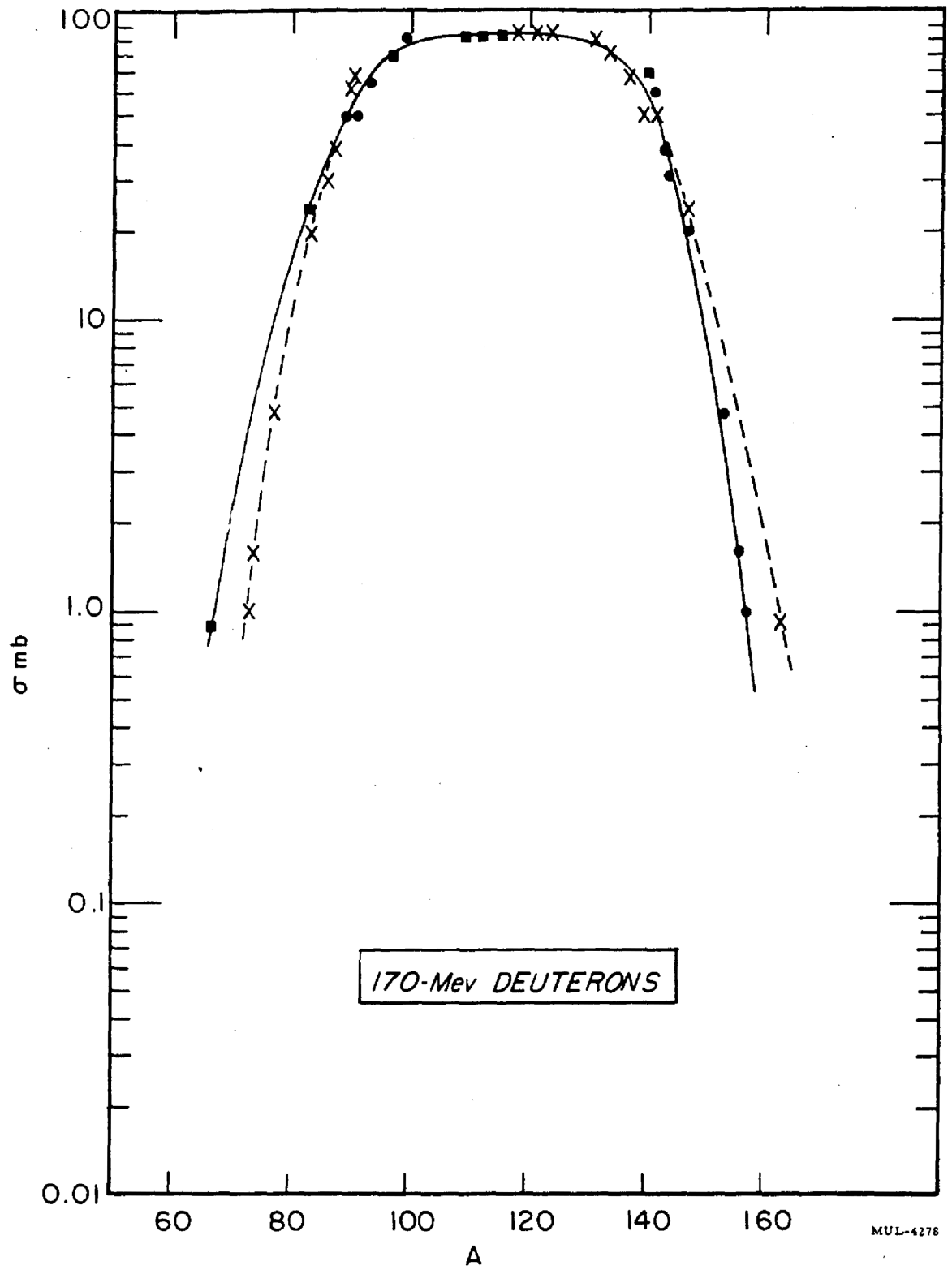
Fig. 2 G. 170-Mev Deuterons
