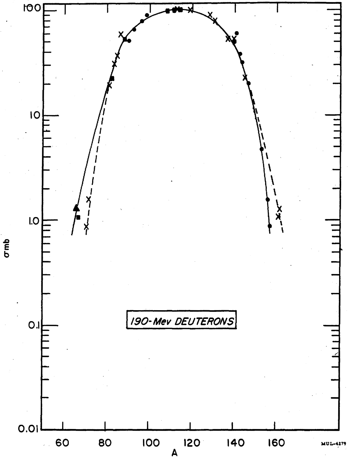
Fig. 2 H. 190-Mev Deuterons
