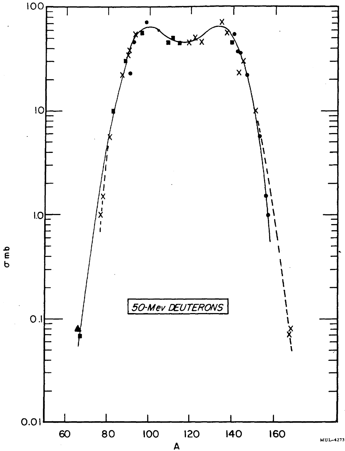
Fig. 2 B. 50-Mev Deuterons
