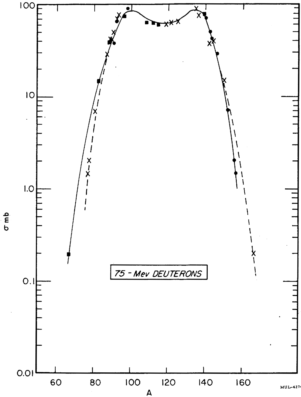
Fig. 2 C. 75-Mev Deuterons
